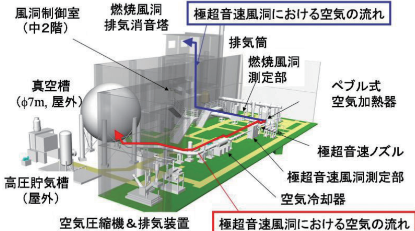
図1 「極超音速高エンタルピー風洞」の概略図：高圧貯気槽にある高圧の気体をペブル式空気加熱器により高温に加熱する。高温の気流で実験する場合は気体をそのまま燃焼風洞測定部に通す。高速の気流で実験をする場合はノズルで真空槽とつなぎ、熱エネルギーを運動エネルギーに変換する。実験で使った超高速流れは、真空槽に排気される。
