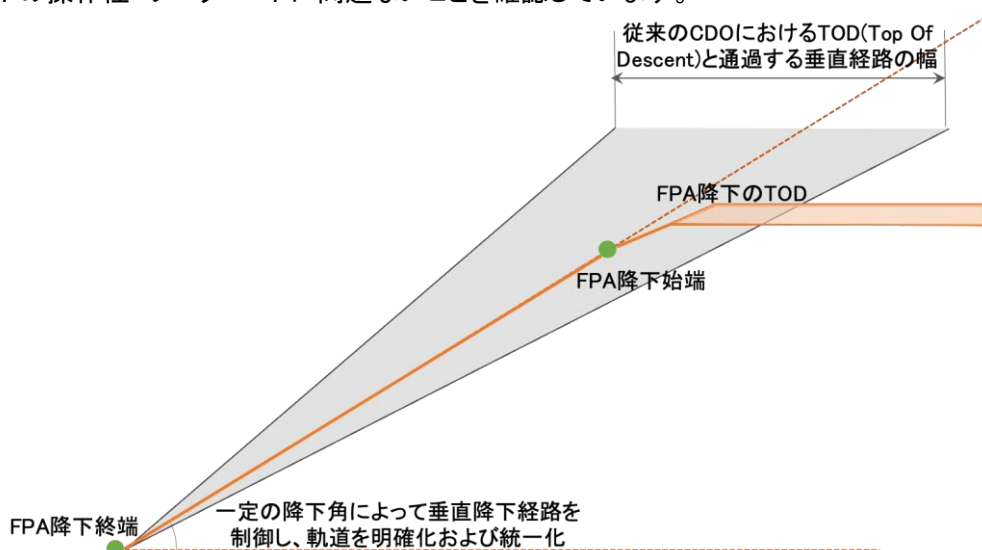
FPA 降下の概念図 (TOD: 水平巡航飛行からの降下開始の点)
