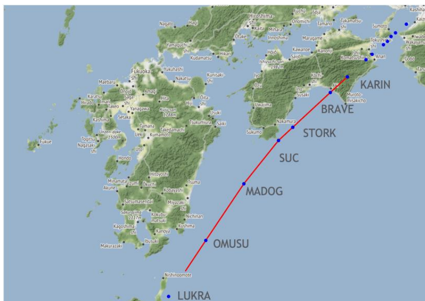
当該実証飛行が FPA 降下を実施した飛行経路
