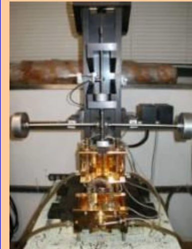
内部摩擦法による構造敏感性の研究
