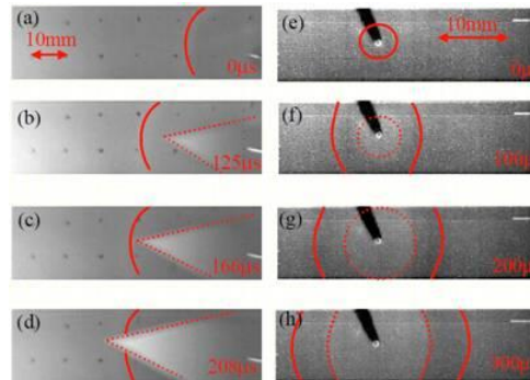
超弾性的に振舞うゴム材料(左)や線形弾性のシャボン玉(右)における高速き裂伝播。実験により、き裂が単一材料でも超音速で進展することがわかった。
